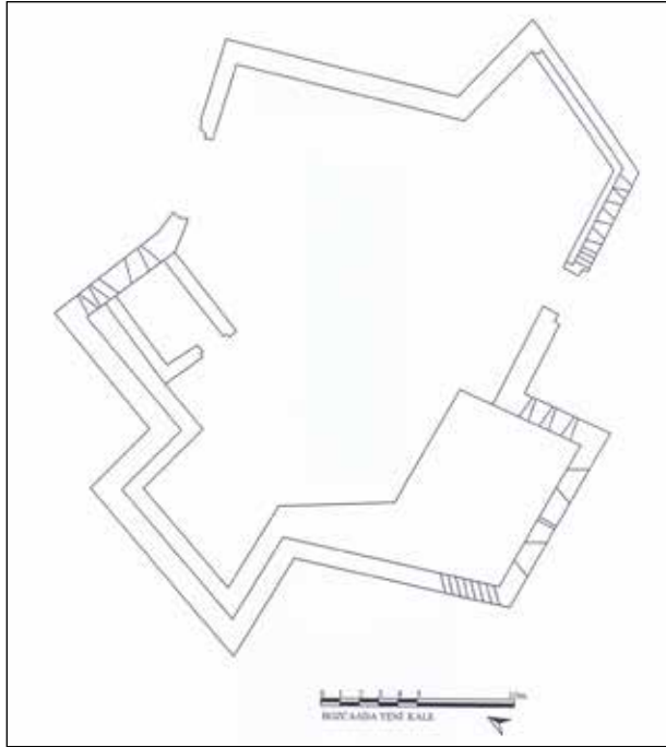
Çizim 12. Bozcaada Yeni Kale planı.
