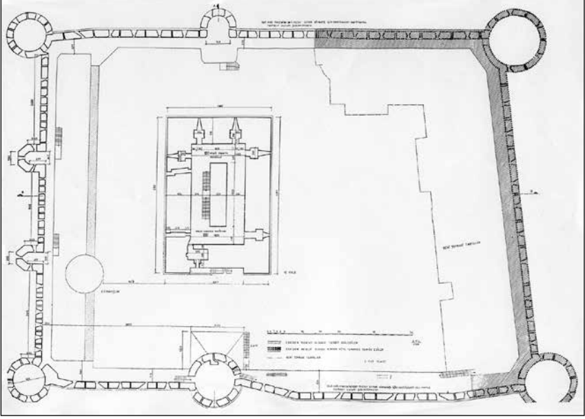
Çizim 3. Kal'a-i Sultâniyye (Çimenlik Kalesi) planı (Ekrem Hakkı Ayverdi'den).
