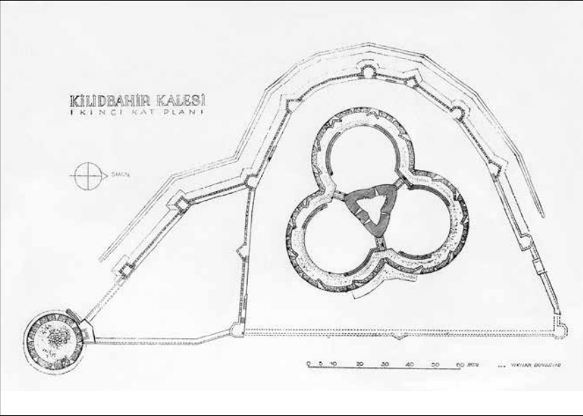
Çizim 4. Kıldü'l-Bahr (Kilitbahir) Kalesi planı (İsmail Utkular'dan).
