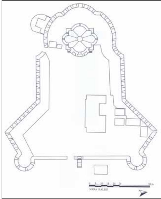
Çizim 8. Nara Kalesi planı.
