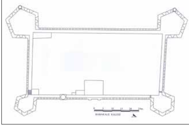
Çizim 7. Hırzû'l-Bahr (Babakale) Kalesi planı.
