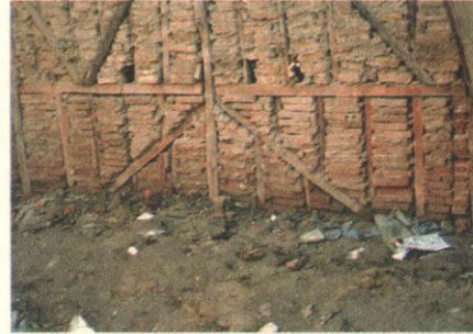
Res. 9 Kerpiç bloklarda Çanakkale seramikleri parçalarının dolgu malzemesi olarak kullanıldığı duvar örgüsü.
