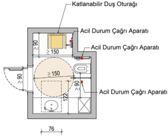
Şekil 12.2.2. Duş Bölümü ve Tuvaletin Olduğu Banyo Örneği
