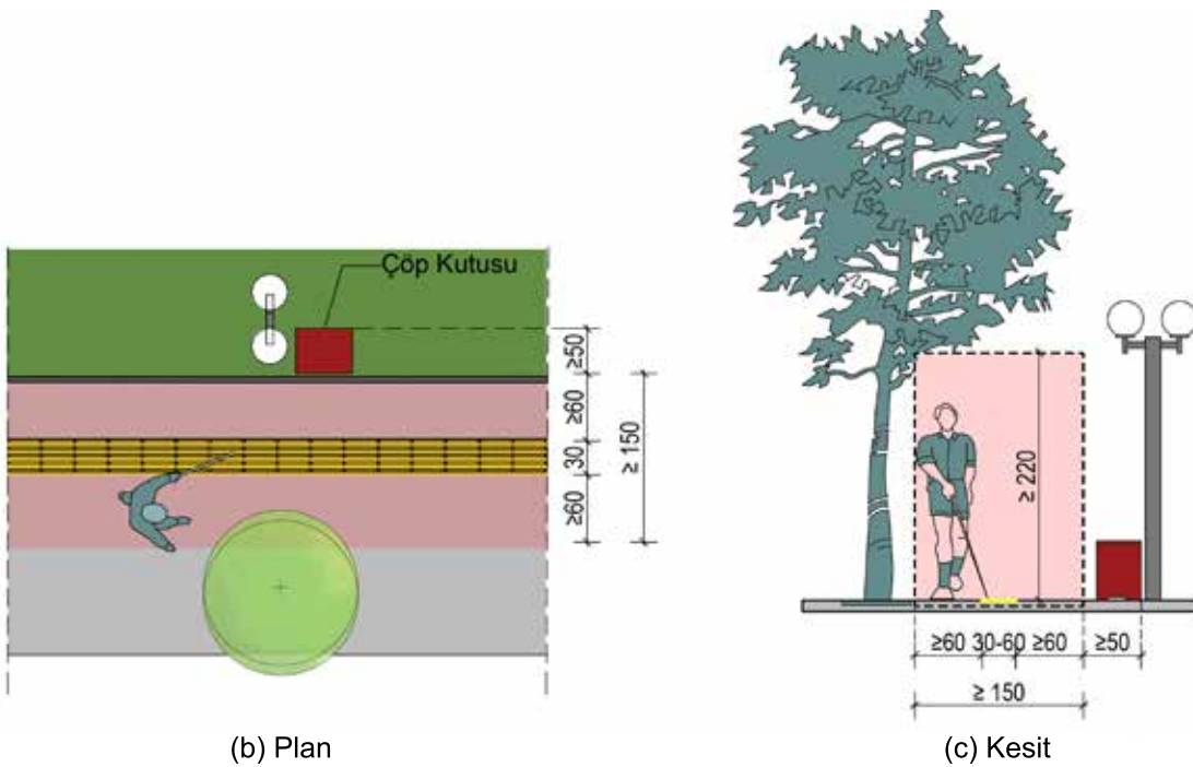
Şekil 11.6. Açık Alanda Kılavuz Yüzey Uygulaması
