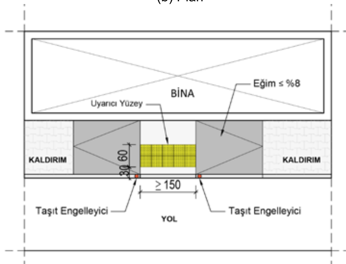
Şekil 2.12. Yola Paralel Kaldırım Rampaları (devam)
