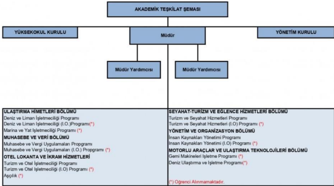
Şekil 9.1 Organizasyon Şeması
