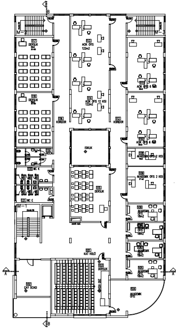
1' KAT PLANI
